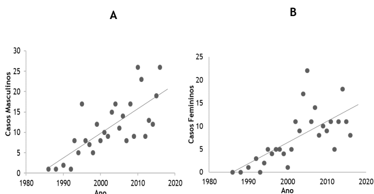
Figura 2. Gráfico de dispersão dos casos e regressão linear, com reta de tendência do sexo masculino (Painel A) e sexo feminino (Painel B)
