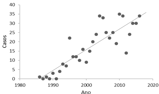
Figura 1 - Casos de HIV/AIDS e reta de tendência. Período de 1986 a 2016. Montes Claros - MG, Brasil.
